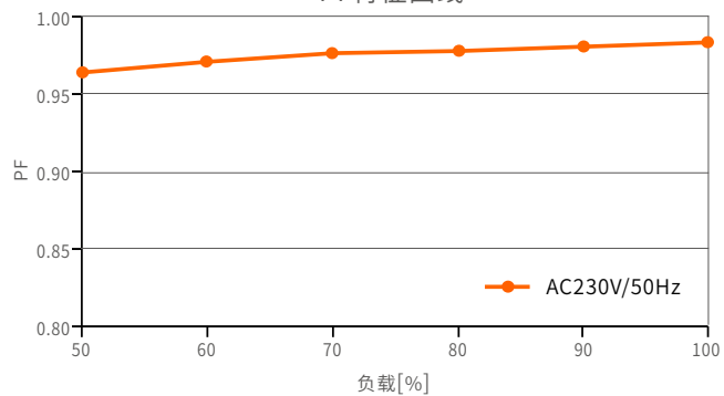
PF特征曲线
