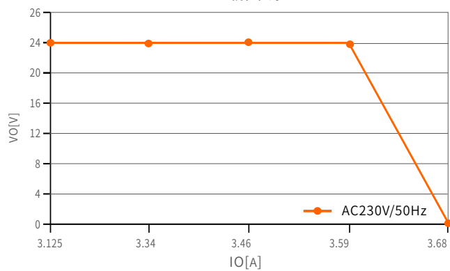
过载曲线
