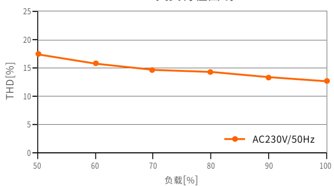
THD失真特征曲线
